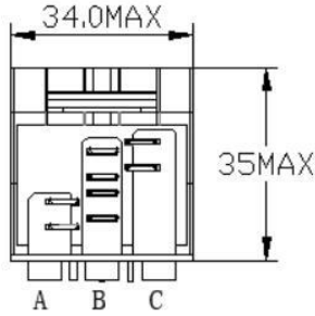
次级正面图
