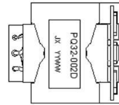
侧面图
